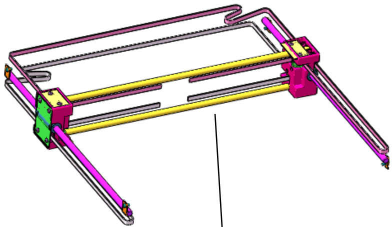
20.204.0193 XY轴套件 X & Y Axis Kit
