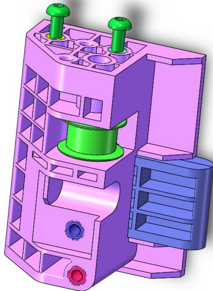
20.205.0114 右前惰轮固定组件 Left Front Idler Fixation Assembly
