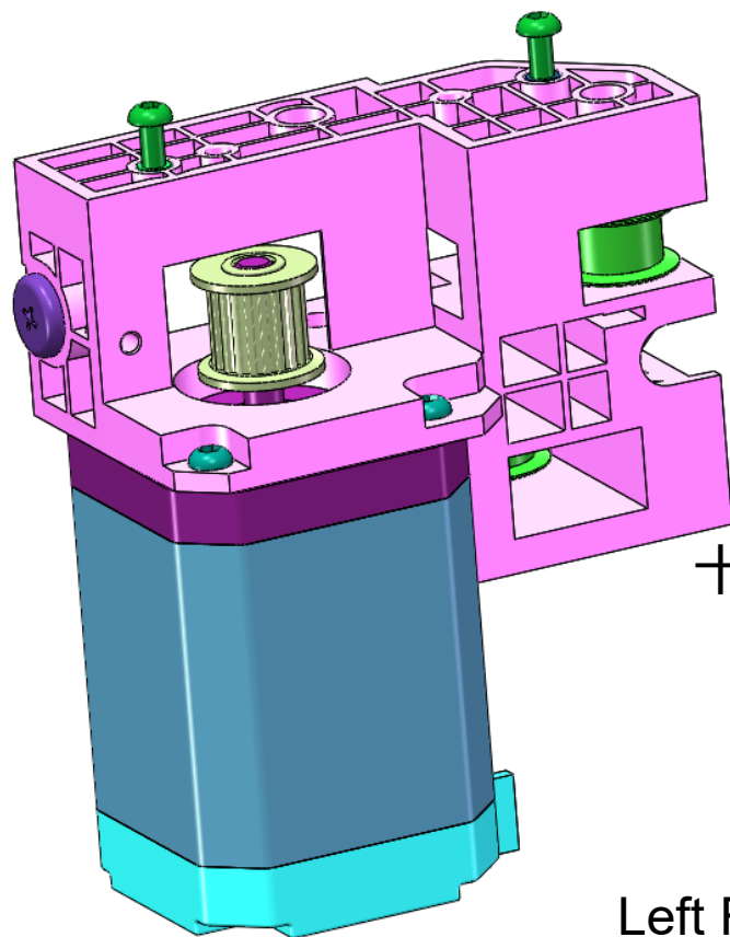
20.205.0112 XY右电机座组件 X & Y Axis Right Motor Base
