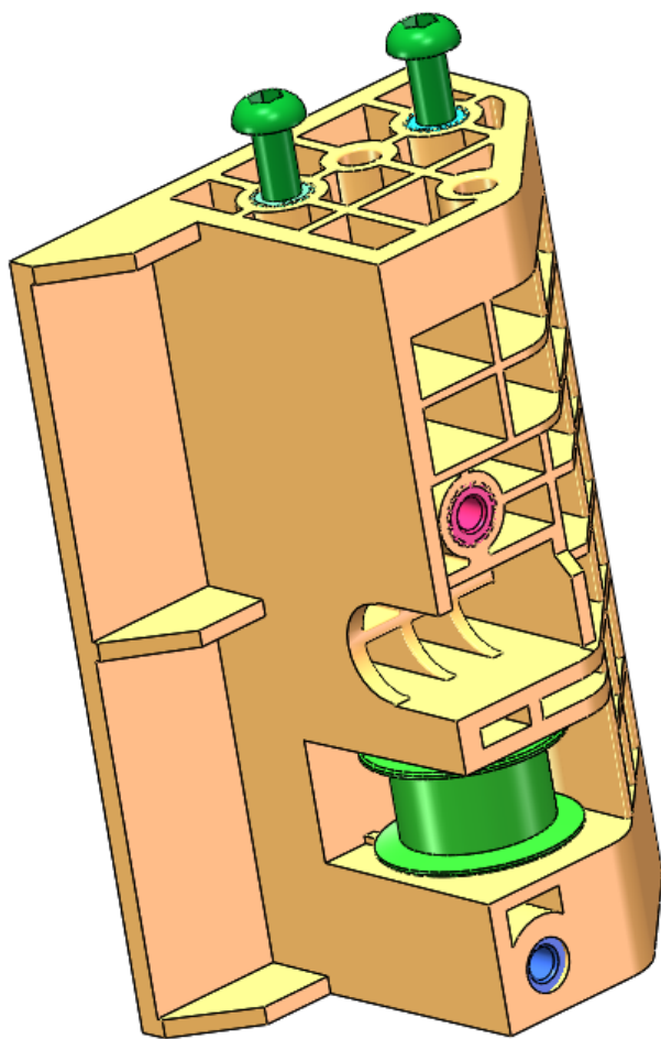
20.205.0113 左前惰轮固定组件 Left Front Idler Fixation Assembly
